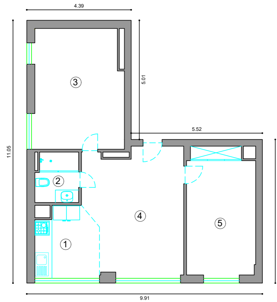
PLANTA PISO 1 - FRAÇÃO C ESC.: 1/100
